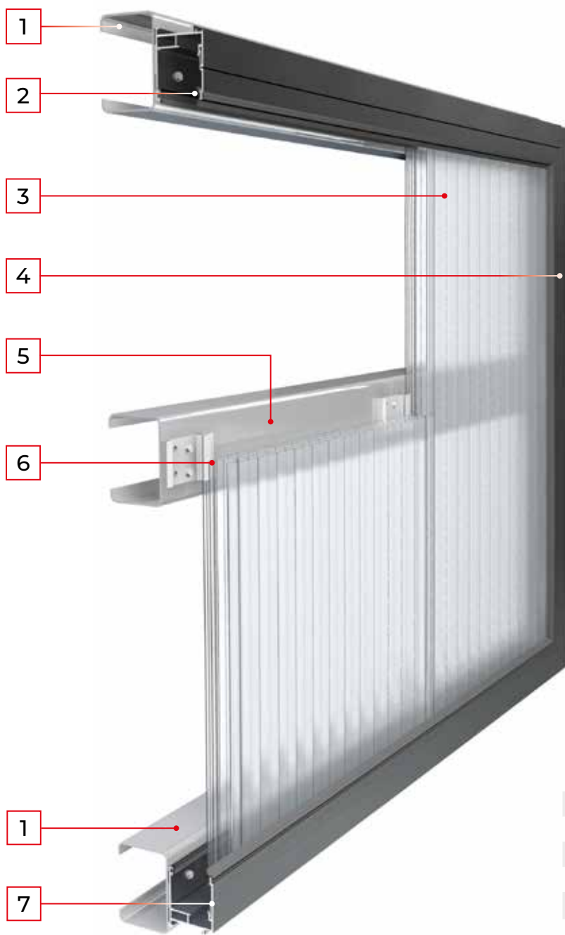
Rys. 1 Konstrukcja naświetla ściennego
